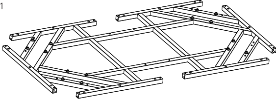
STRUCTURE ESTRUCTURA
