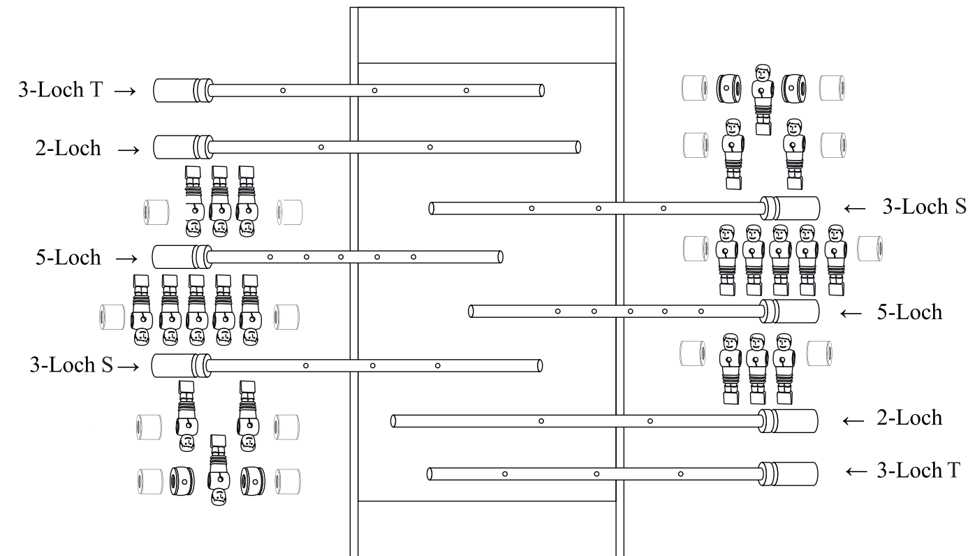
Abb: Modell Coupé (bei Modell Evolution sind alle 3-Loch-Stangen identisch)
